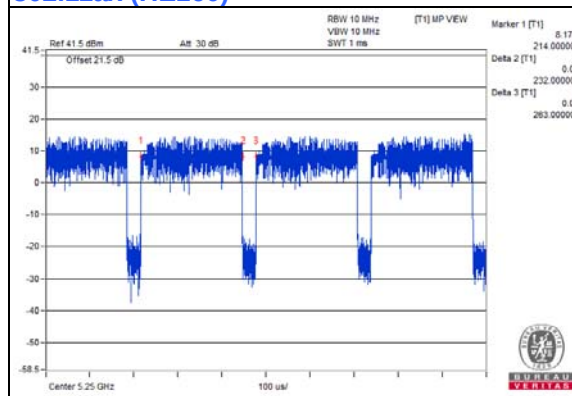
802.11ax (HE160)
