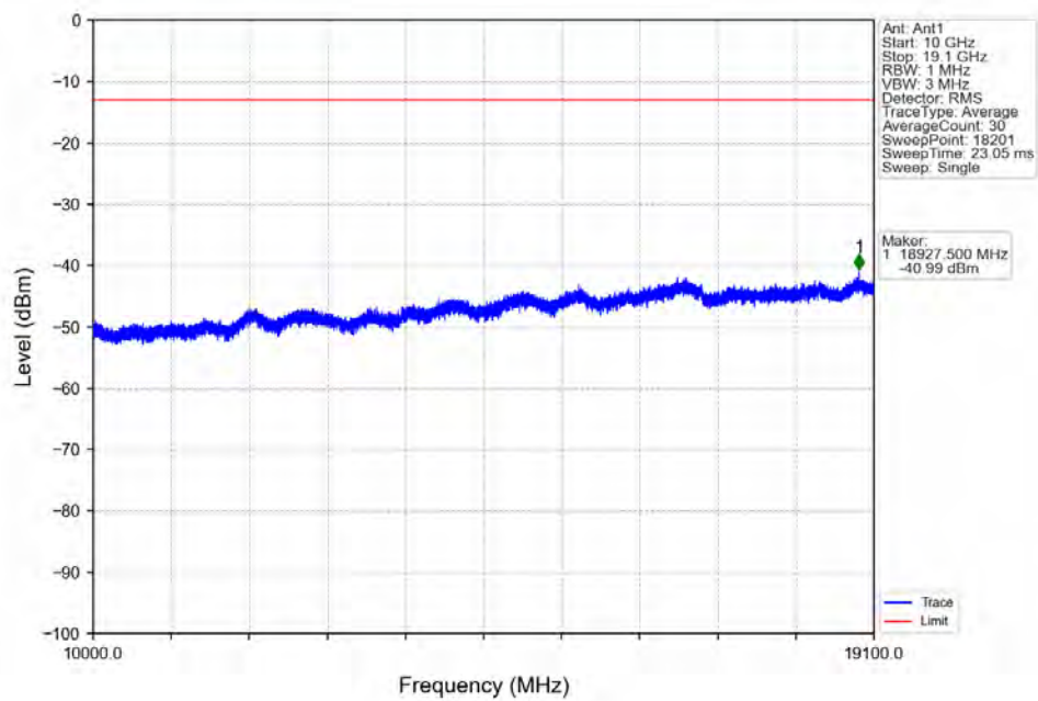
Band2_3MHz_QPSK_HCH_1908.5MHz_RB_1_14_NTNV
