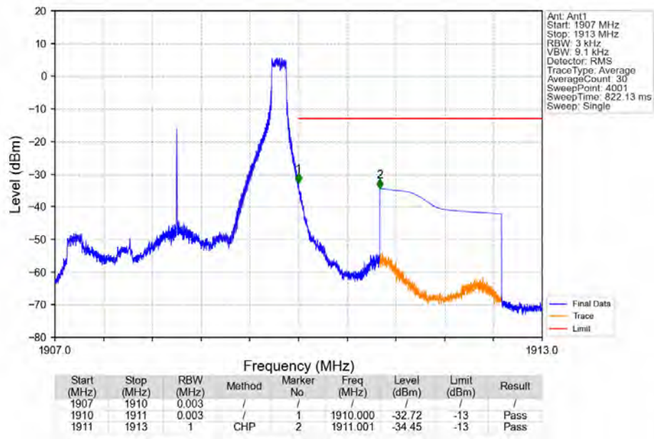
Band2_3MHz_QPSK_HCH_1908.5MHz_RB_1_14_NTNV
