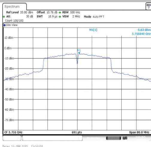
11N40SISO-Ant1-5755-PASS
