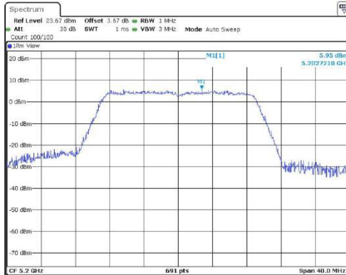
11N20MIMO_Ant1_5200
