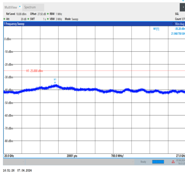
Band7_20MHz_QPSK_20850_1RB#0_20000~27000_20000~27000
