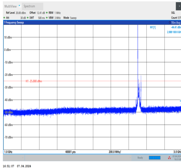
Band7_20MHz_QPSK_20850_1RB#0_1000~3000_1000~3000
