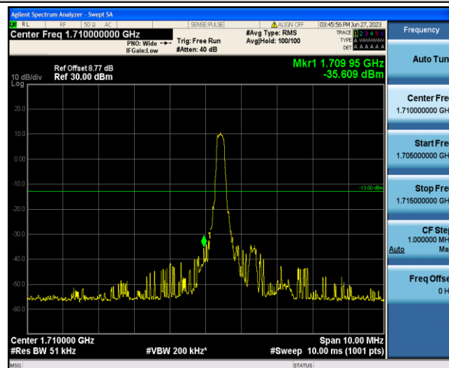
Band4-3MHz-QPSK-19965-1-0-Low--35.61-PASS
