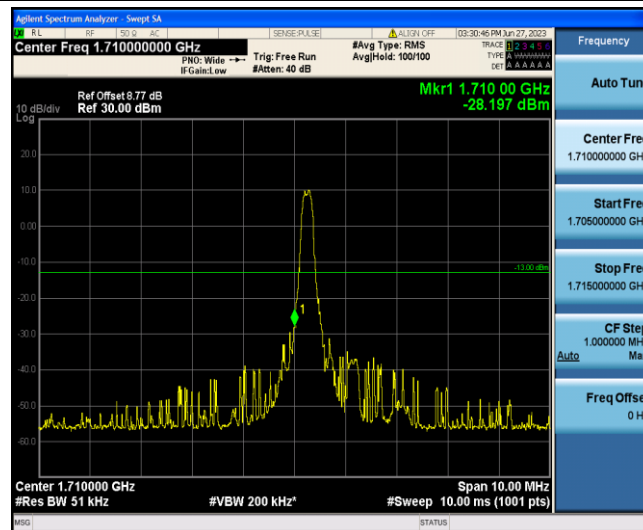
Band4-1.4MHz-QPSK-19957-1-0-Low--28.20-PASS
