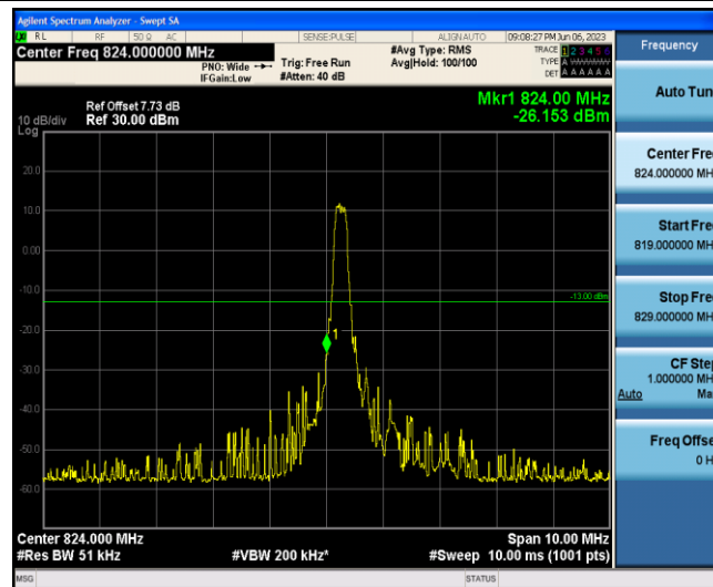
Band5-1.4MHz-QPSK-20407-1-0-Low--26.15-PASS
