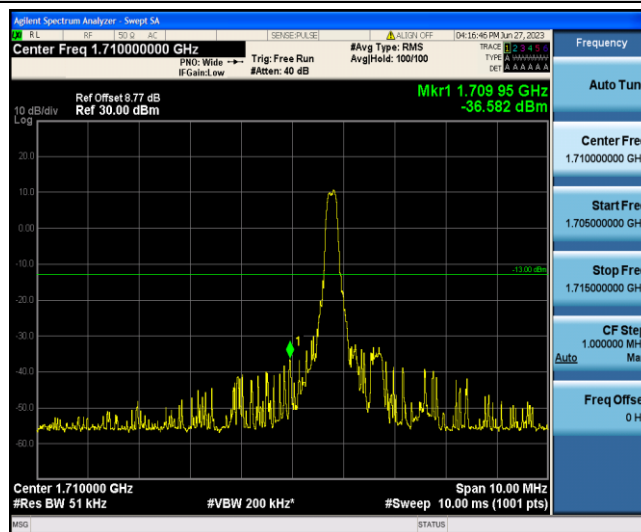
Band4-10MHz-16QAM-20000-1-0-Low--36.58-PASS
