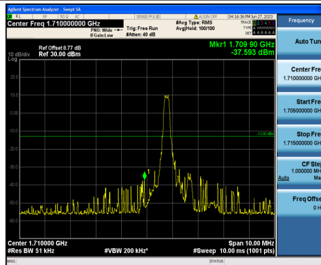
Band4-10MHz-QPSK-20000-1-0-Low--37.59-PASS
