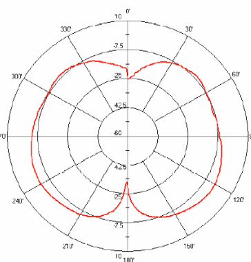
2.4 GHz E-Plane Horizontal
