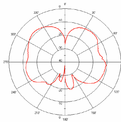
2.4 GHz H-Plane Vertical
