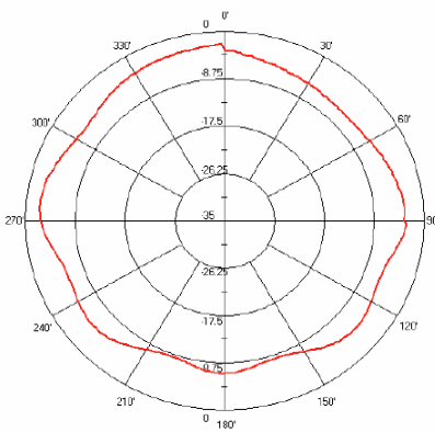
2.4 GHz H-Plane Horizontal
