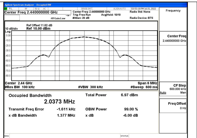
Test Mode:GFSK (LE 2Mbps)
