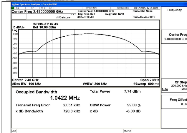
Test Mode:GFSK (LE 1Mbps)
