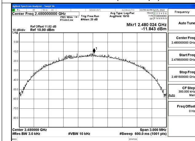
Test Mode:GFSK (LE 2Mbps)
