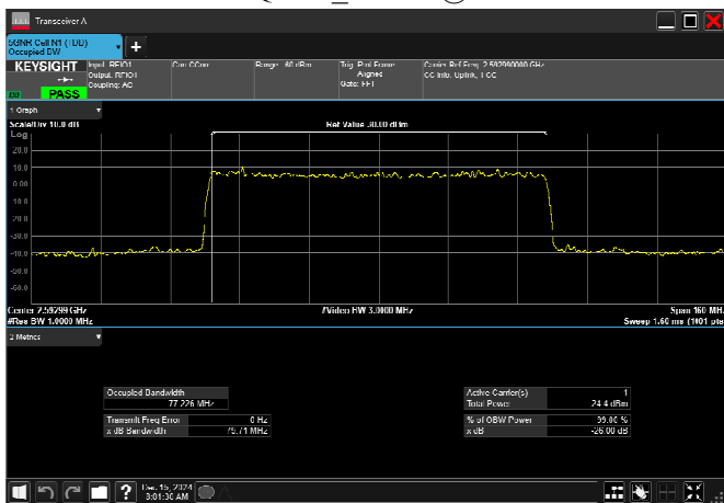
n41_80MHz_30kHz_2592.99MHz_DFT-s-OFDM QPSK_RB216@0
