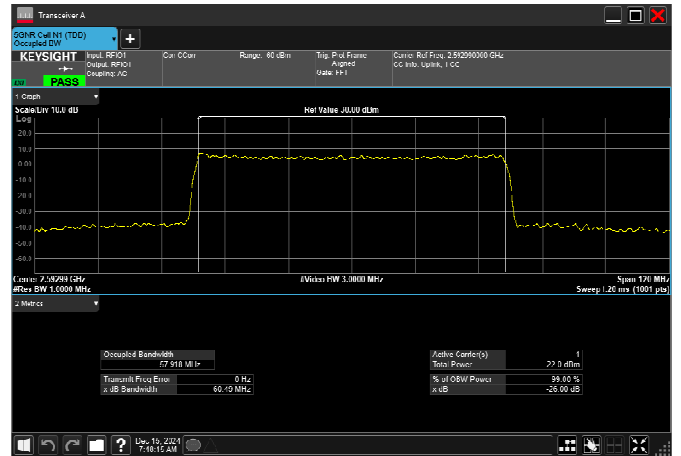
n41_80MHz_30kHz_2592.99MHz_DFT-s-OFDM \pi/2 BPSK_RB216@0
