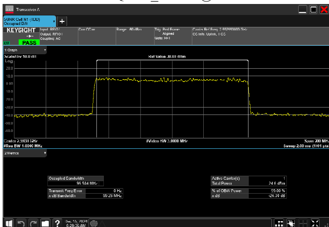
n41_100MHz_30kHz_2592.99MHz_DFT-s-OFDM 16 QPSK_RB270@0
