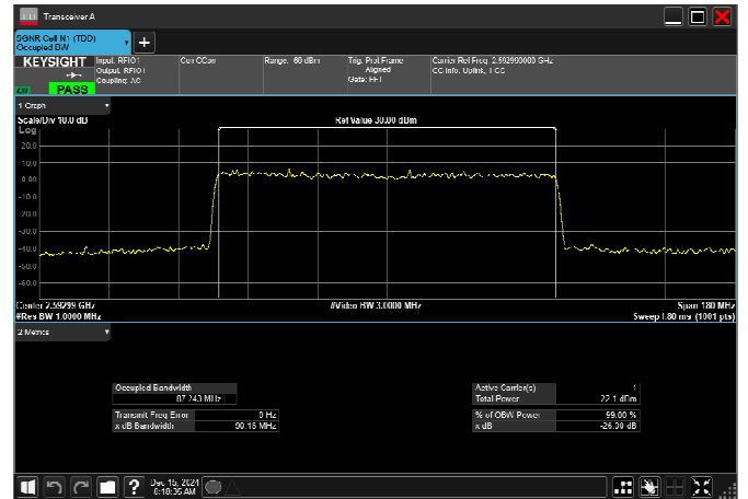
n41_100MHz_30kHz_2592.99MHz_DFT-s-OFDM \pi/2 BPSK_RB270@0
