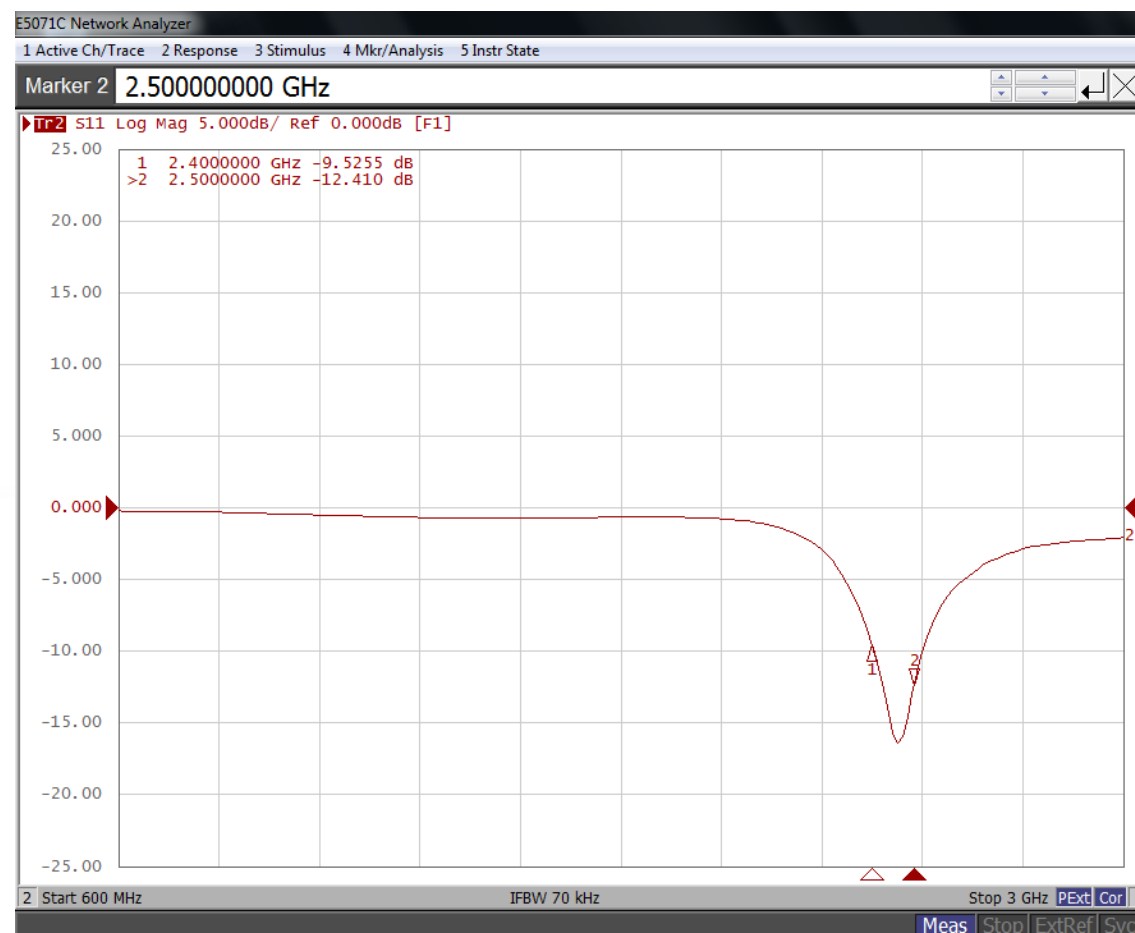
S-Parameter Test
