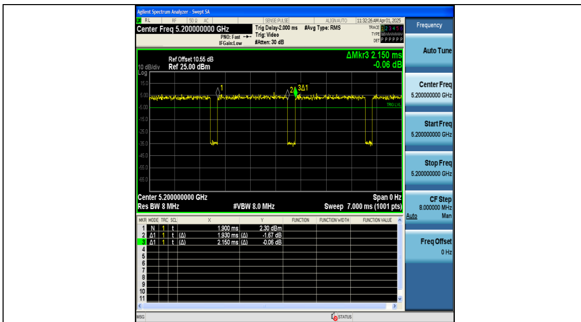
NTNV-11AC20MIMO-Ant1-5200
