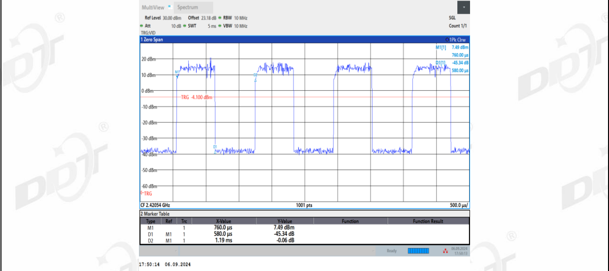
11AX20MIMO_Ant2_2412_52Tone_RU37
