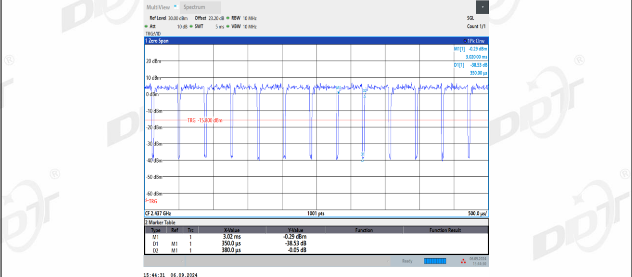
11N40MIMO_Ant2_2437
