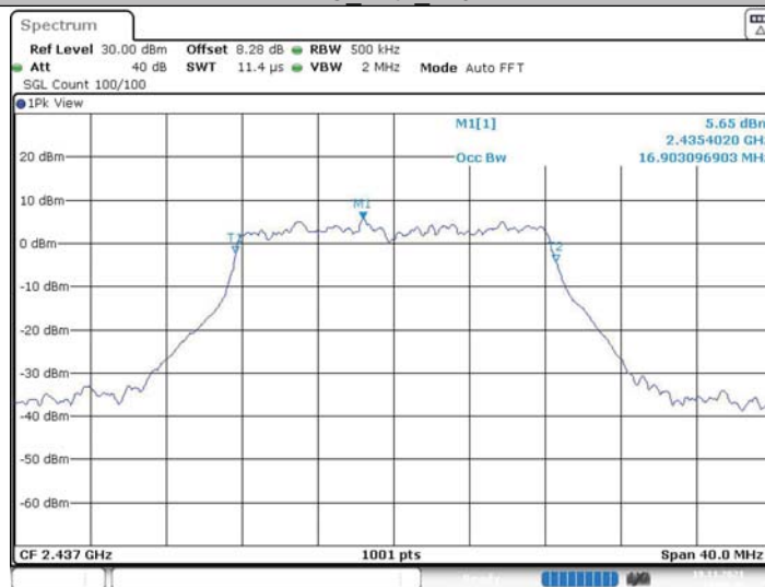
11G_Ant2_2437
