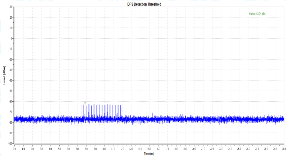
11AC80_5290_Type3
