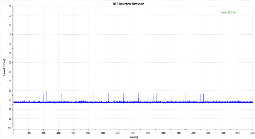
11N40_5510_Type6
