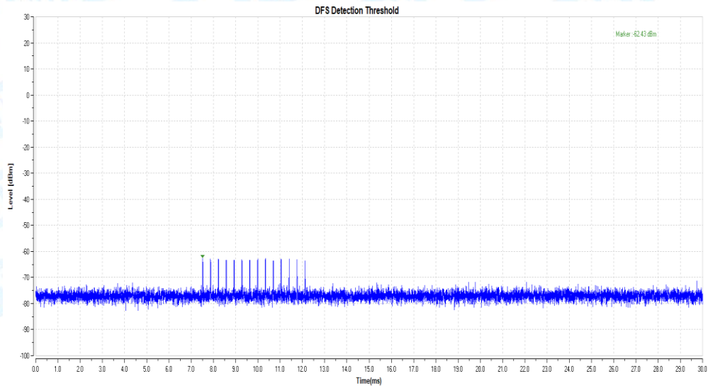
11N40_5510_Type5
