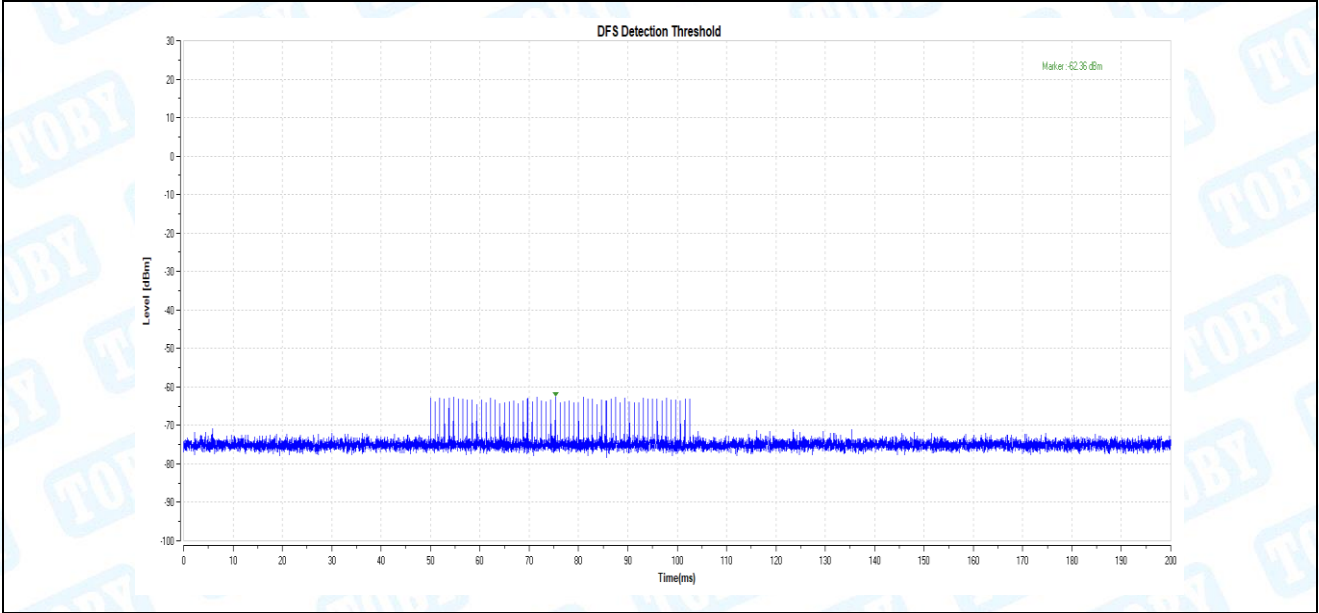
11N40_5510_Type2
