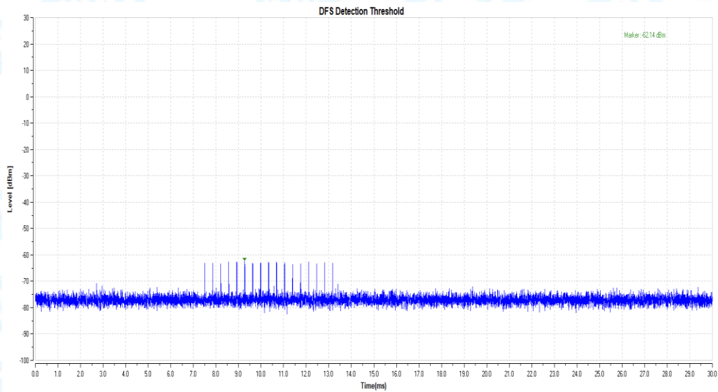
11N40_5510_Type4
