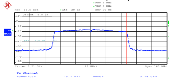
802.11ac(HT80)
