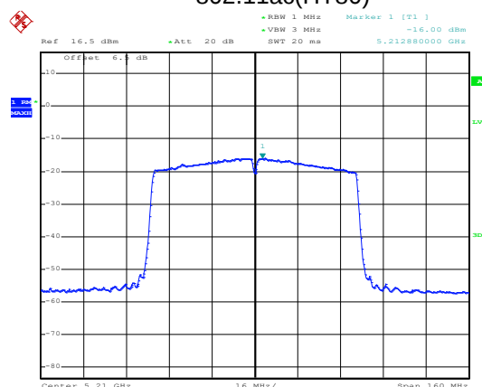
802.11ac(HT80)
