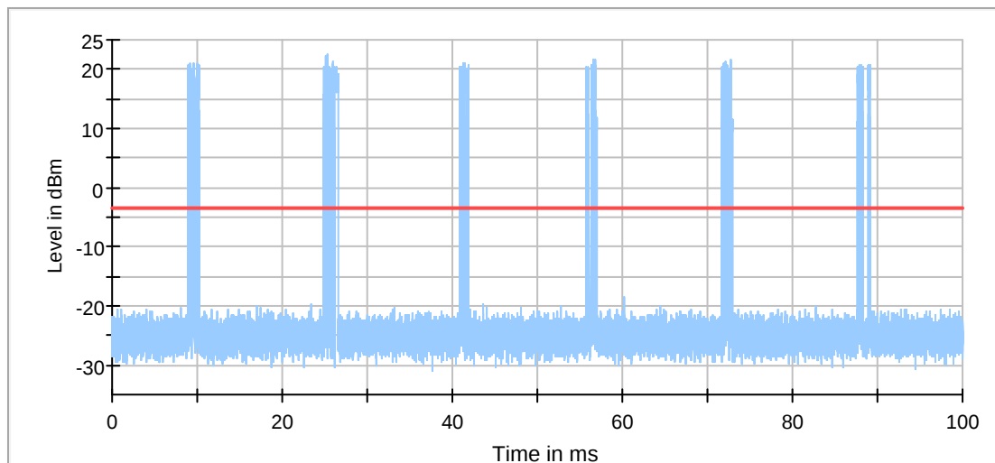
802.11a 5260MHz
