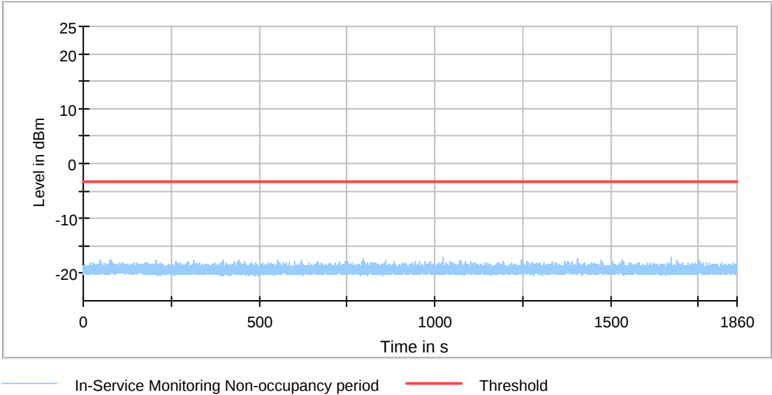
802.11a 5260MHz
