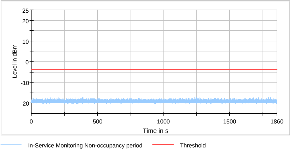
802.11n HT40 5270MHz
