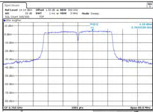
UNII-3 / 802.11ac VHT40 / 5 755 MHz
