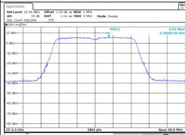
UNII-2C / 802.11ac VHT20 / 5 500 MHz
