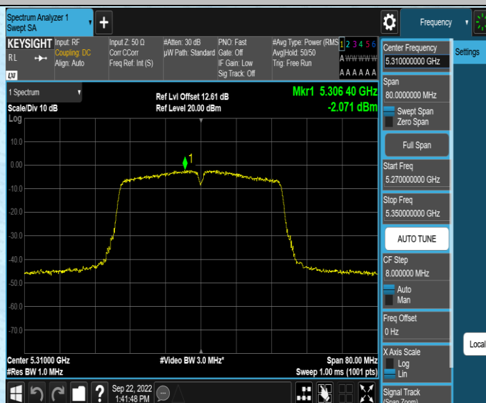
11AC40MIMO_Ant1_5310
