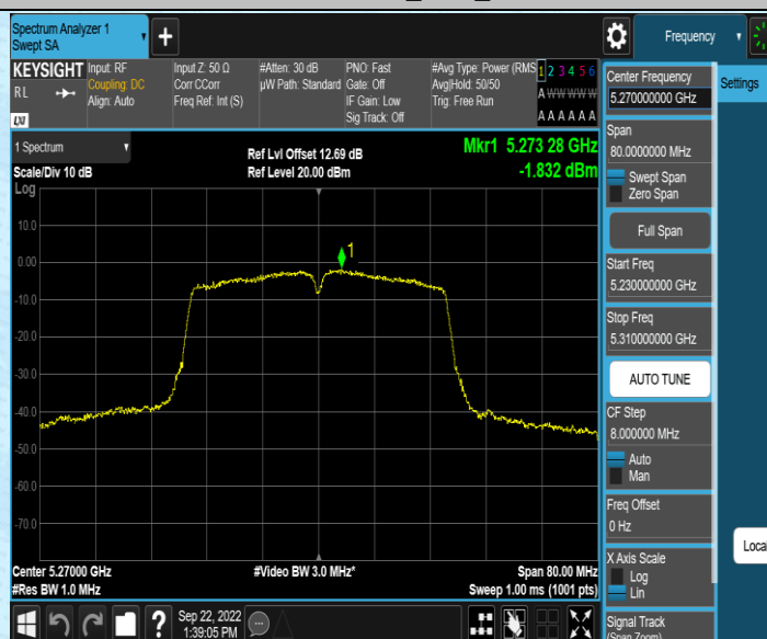
11AC40MIMO_Ant1_5270
