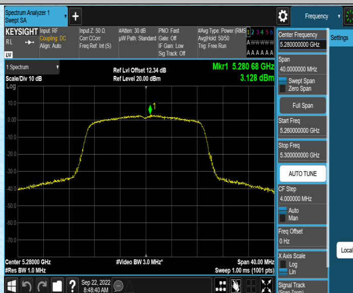
11N20SISO_Ant2_5280
