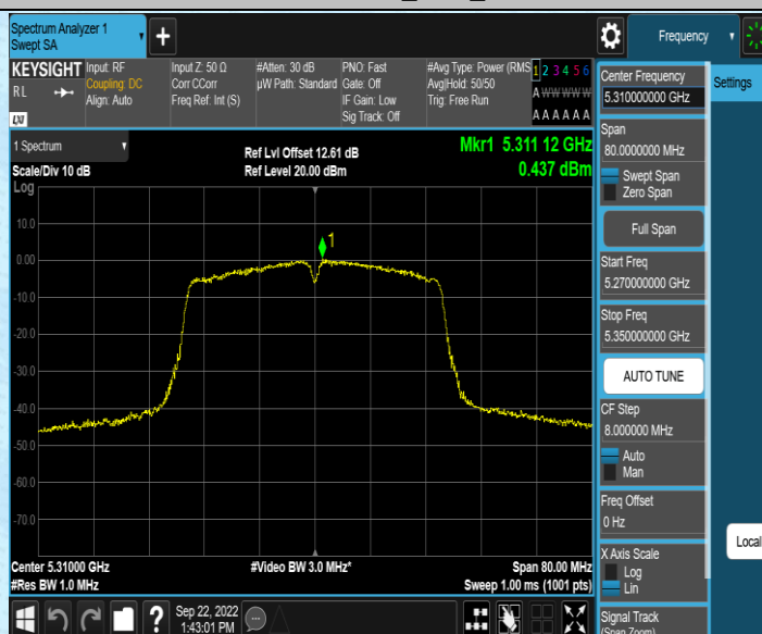
11AC40MIMO_Ant2_5310
