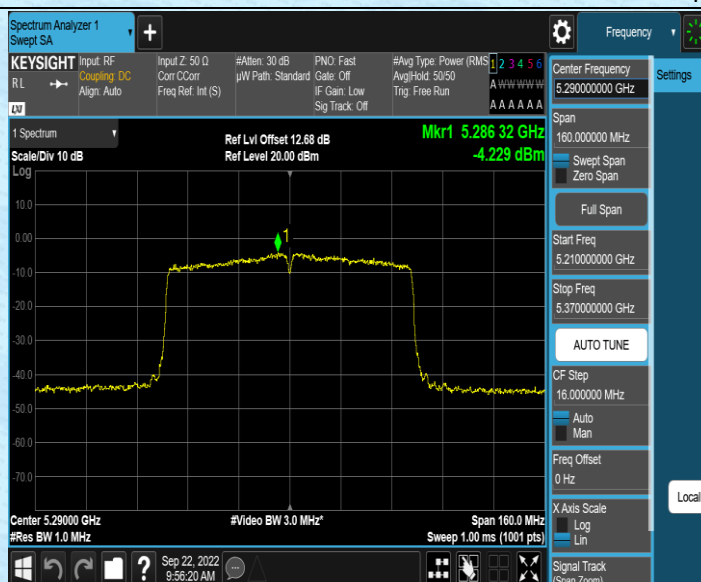
11AC80SISO_Ant2_5290
