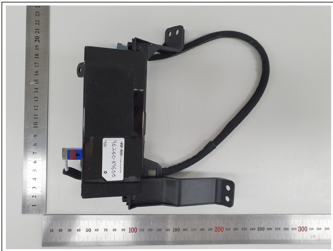
<LTE Rx Antenna>
