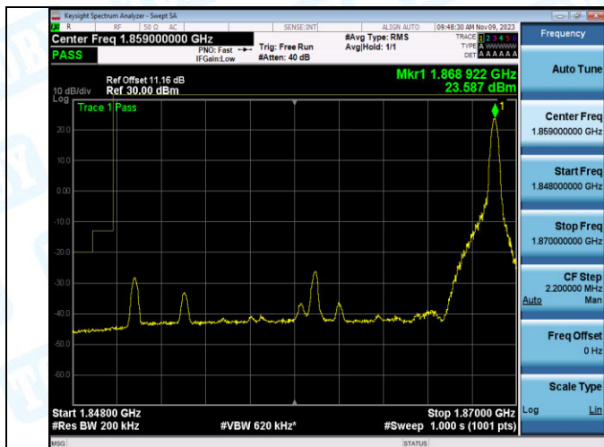
Band2_20MHz_QPSK_18700_1RB#99
