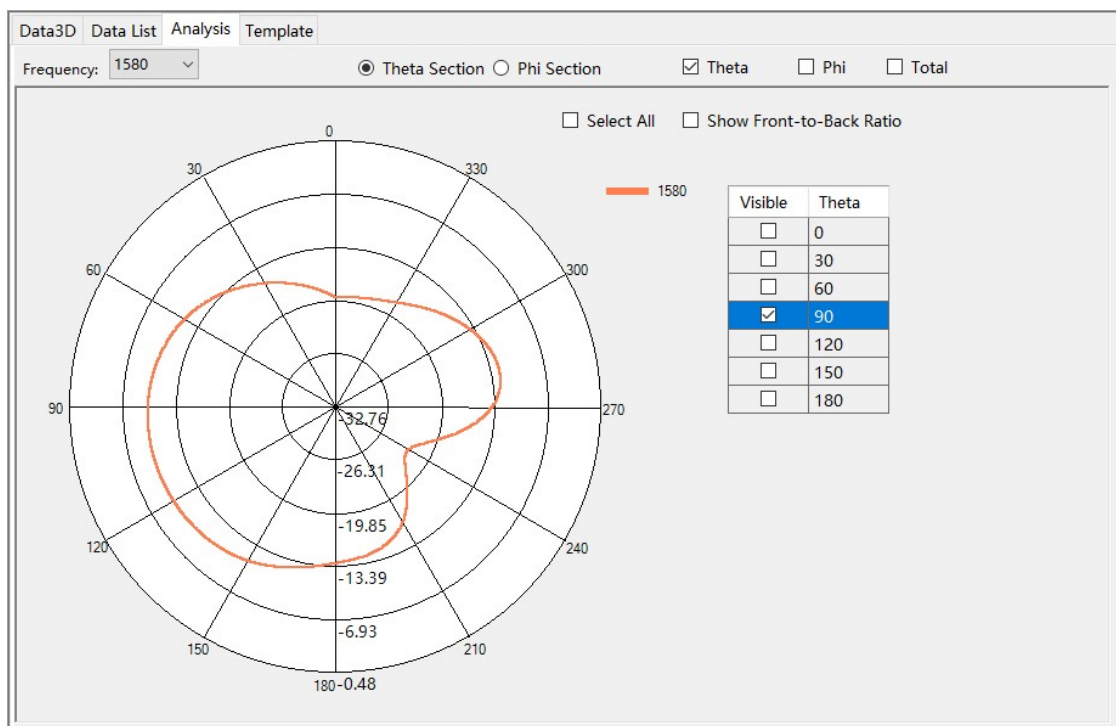
GPS Theta=90deg
