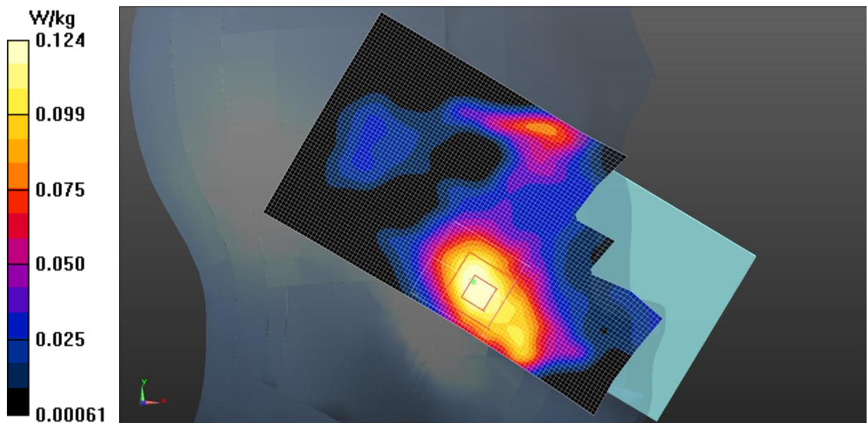
Fig.9 WCDMA 1700
