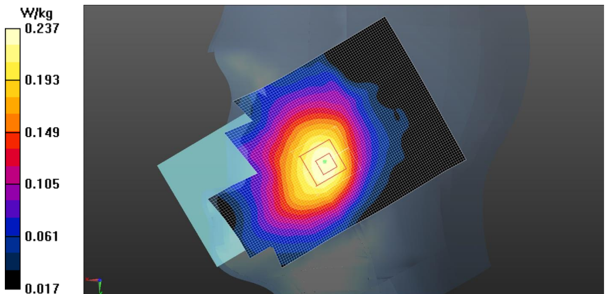
Fig.5 WCDMA 850
