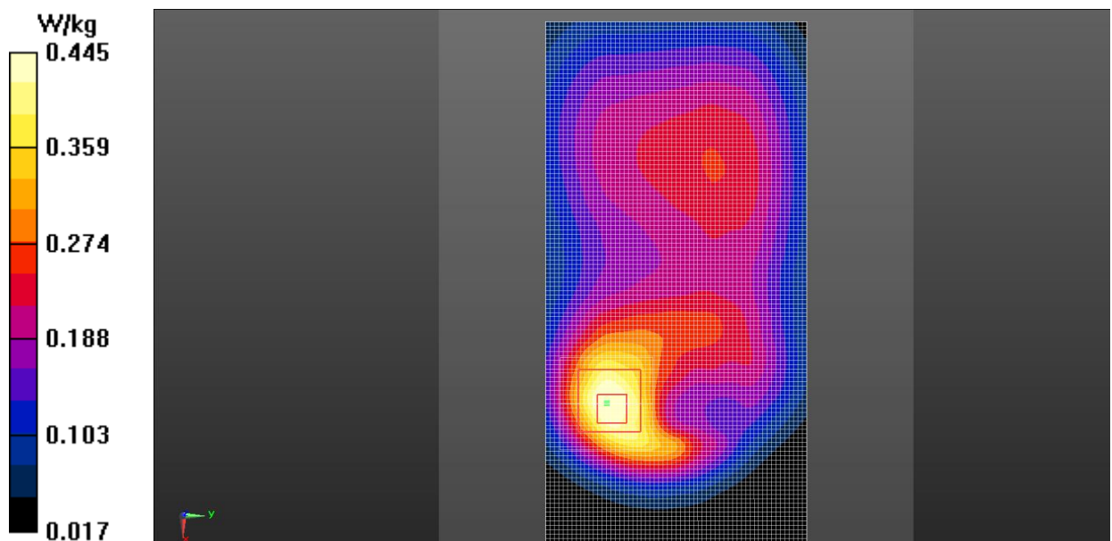
Fig.6 WCDMA 850
