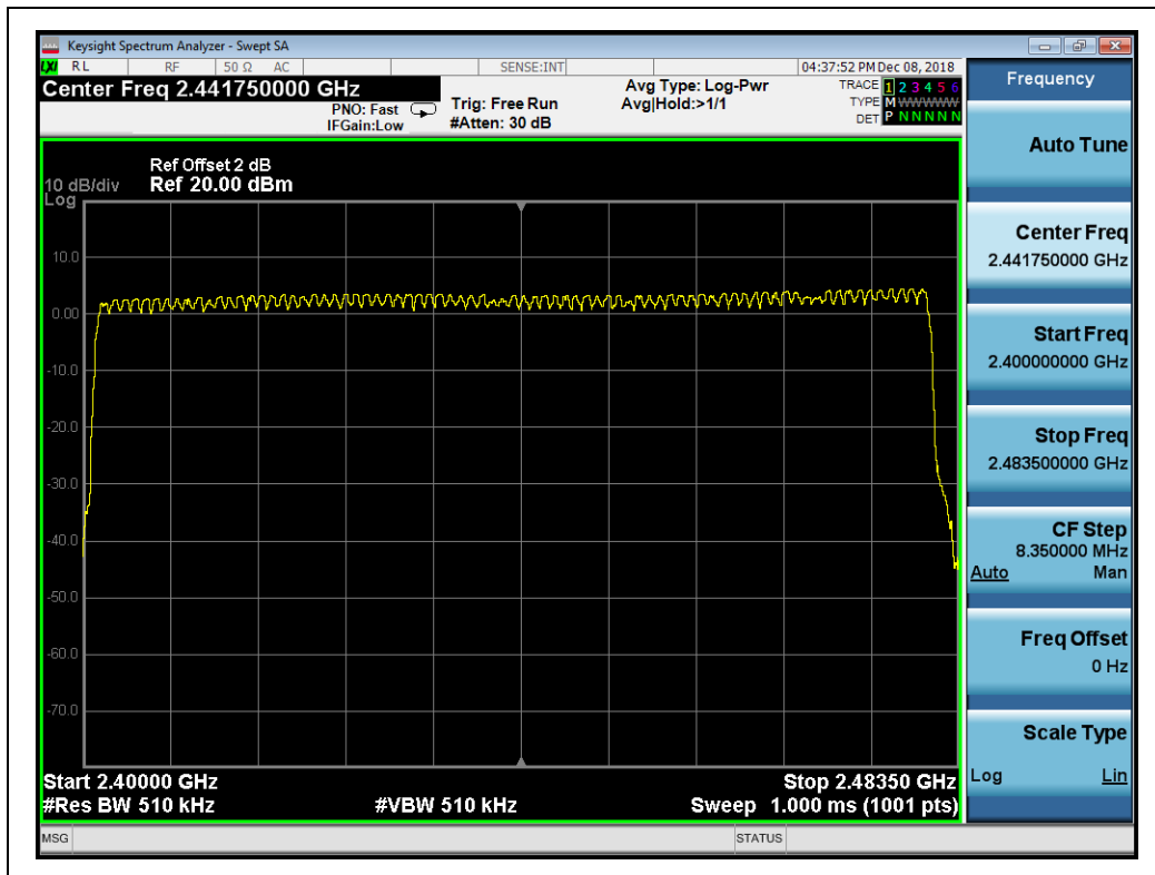
( \pi/4 -DQPSK)
