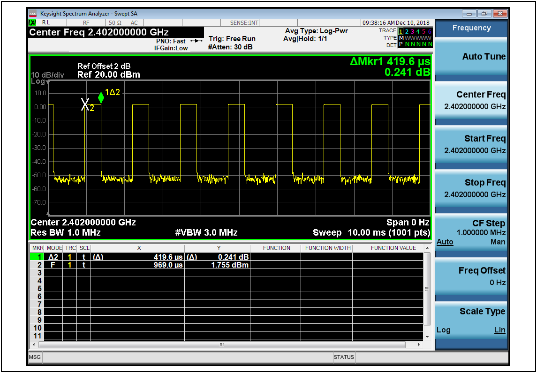
(DH1_2402MHz, GFSK)
