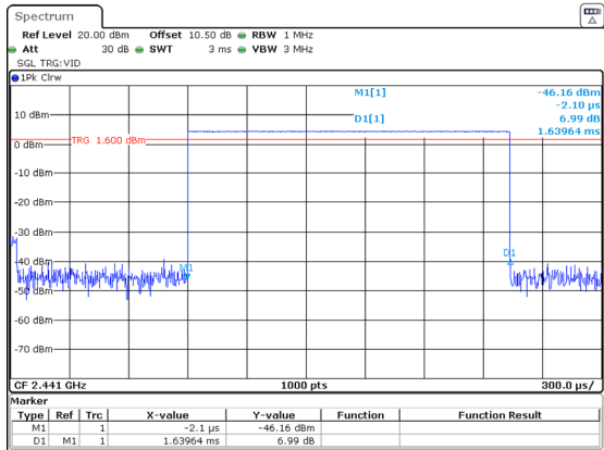
DH3_Hopping 1.640ms
