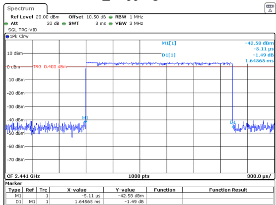
2DH3_Hopping 1.646ms
