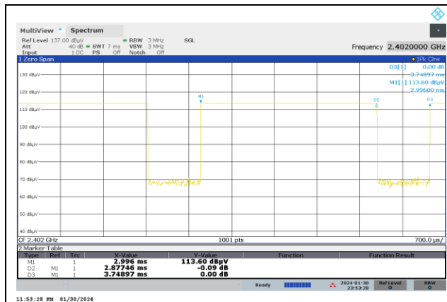
BT GFSK
