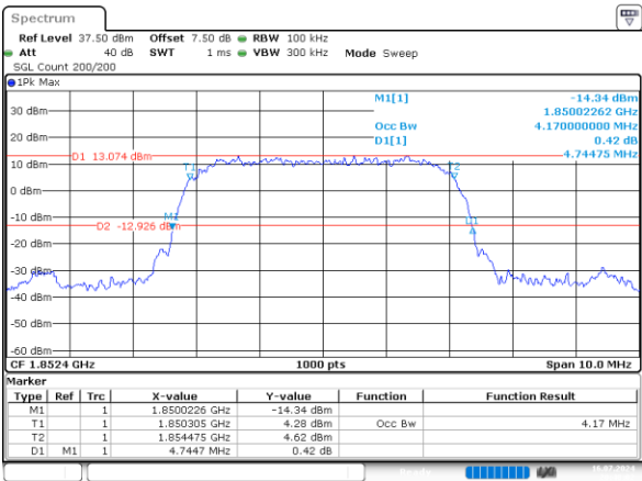
HSDPA_Low_Subtest1 4.170MHz
