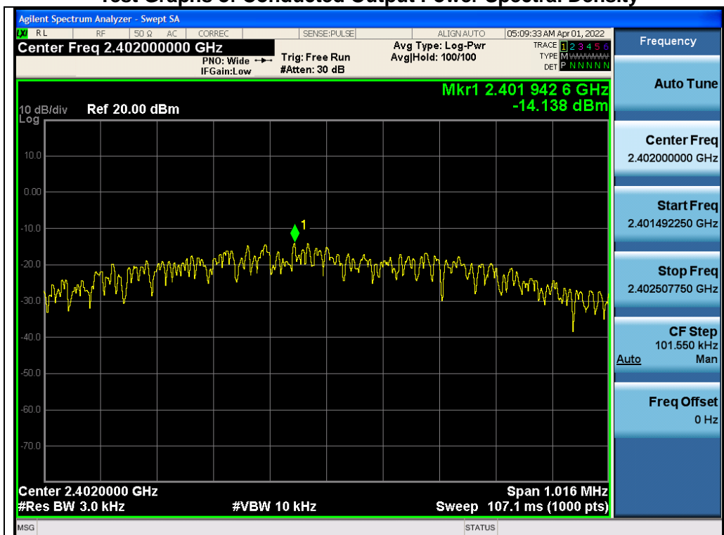
Test_Graph_LE1M_ANT2_2402_1Mbps_PSD
