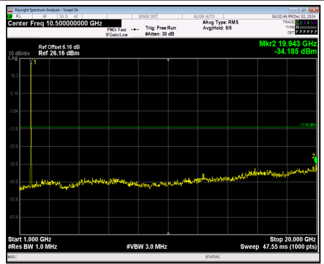
Band66-20MHz-QPSK-132322-1RB#0-Range2:1000~20000MHz
