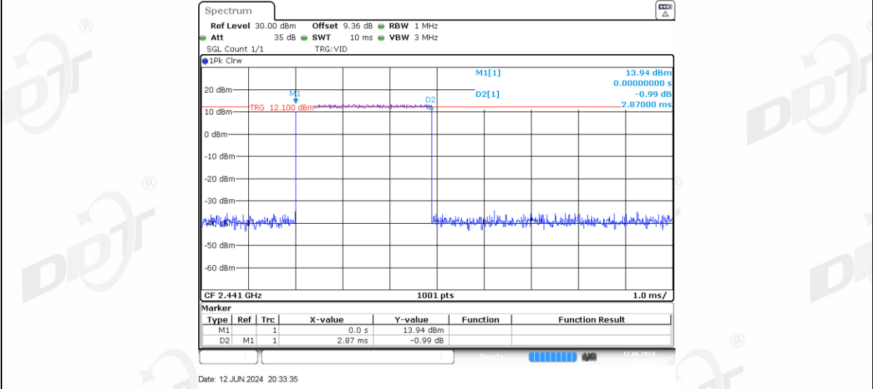
3DH5_Right side_Hop
