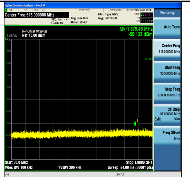
BLE 1M-Ant1-2480-30~1000-PASS
