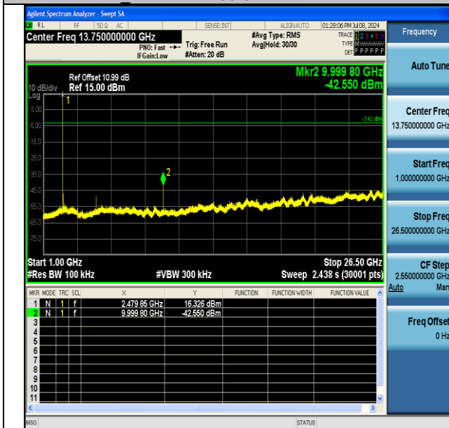
BLE 1M-Ant1-2480-1000~26500-PASS
