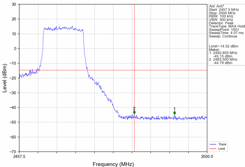
10M_HCH_2467.5MHz_Ant7_NTNV
