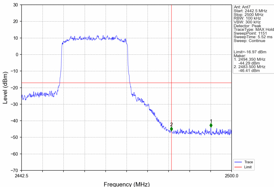
20M_HCH_2462.5MHz_Ant7_NTNV
