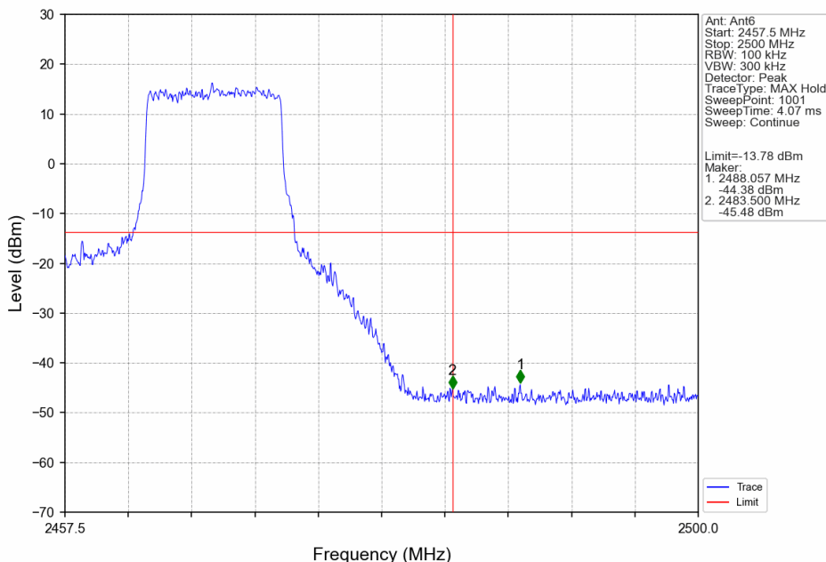
10M_HCH_2467.5MHz_Ant6_NTNV
