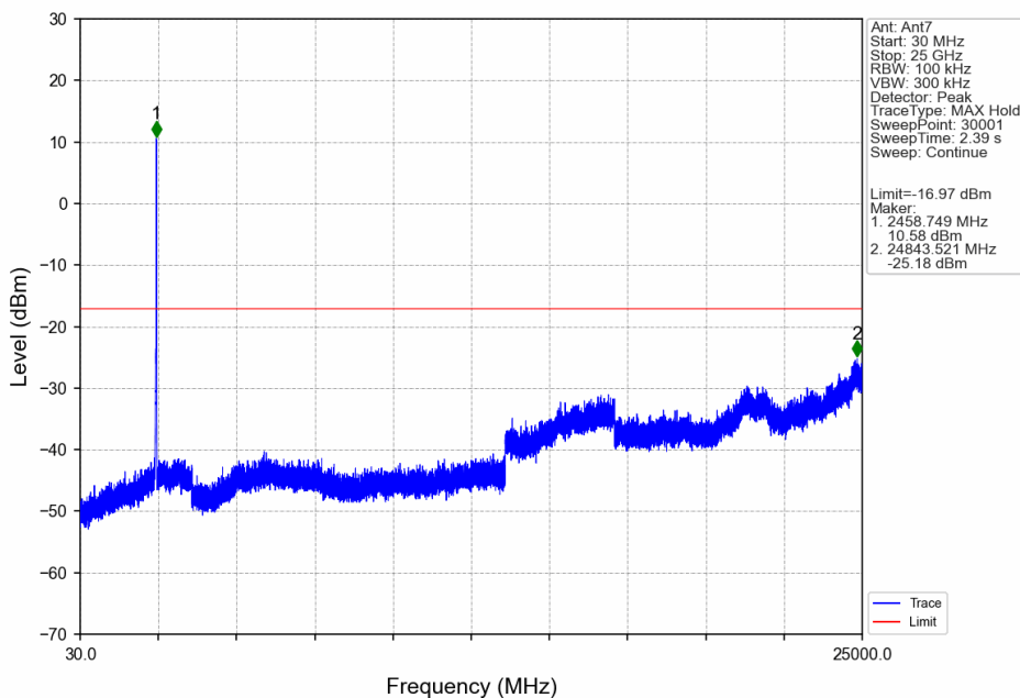
20M_HCH_2462.5MHz_Ant7_NTNV
