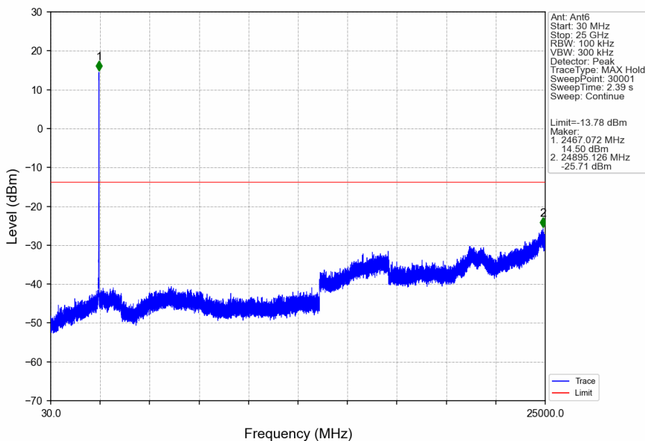
10M_HCH_2467.5MHz_Ant6_NTNV
