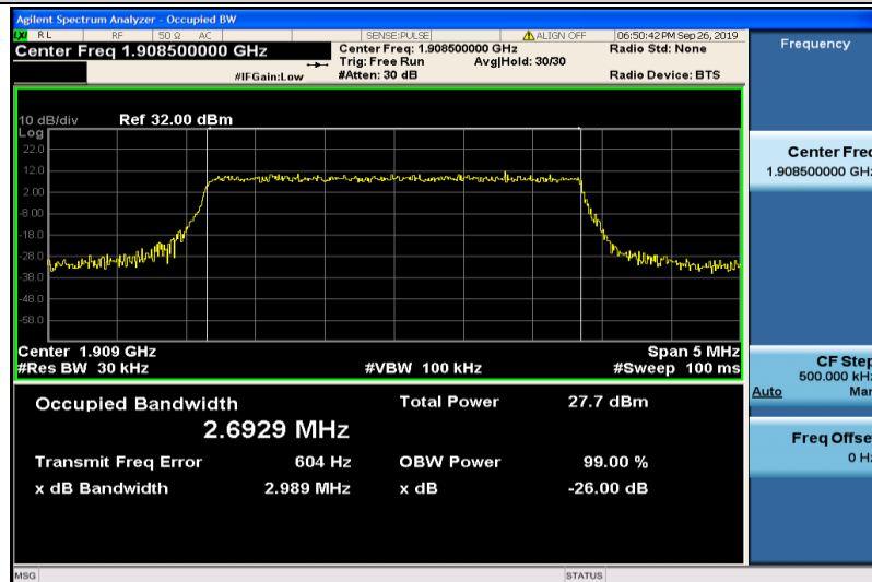
Band2-3MHz-QPSK-19185-15RB#0-2.6929
