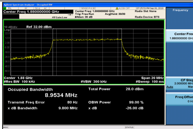
Band2-10MHz-QPSK-18900-50RB#0-8.9534
