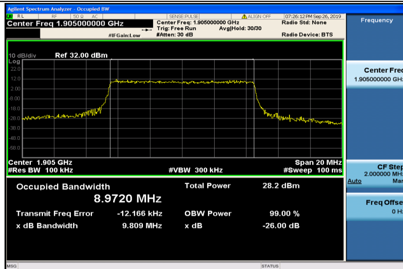
Band2-10MHz-QPSK-19150-50RB#0-8.9720
