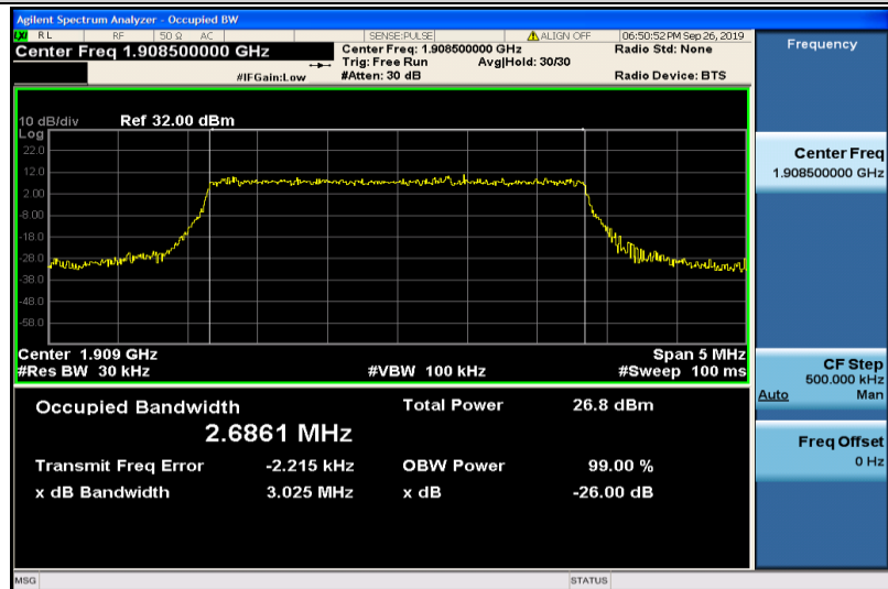
Band2-3MHz-16QAM-19185-15RB#0-2.6861
