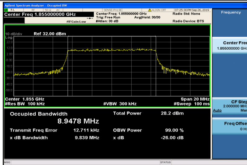
Band2-10MHz-QPSK-18650-50RB#0-8.9478
