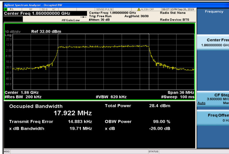
Band2-20MHz-QPSK-18700-100RB#0-17.922
