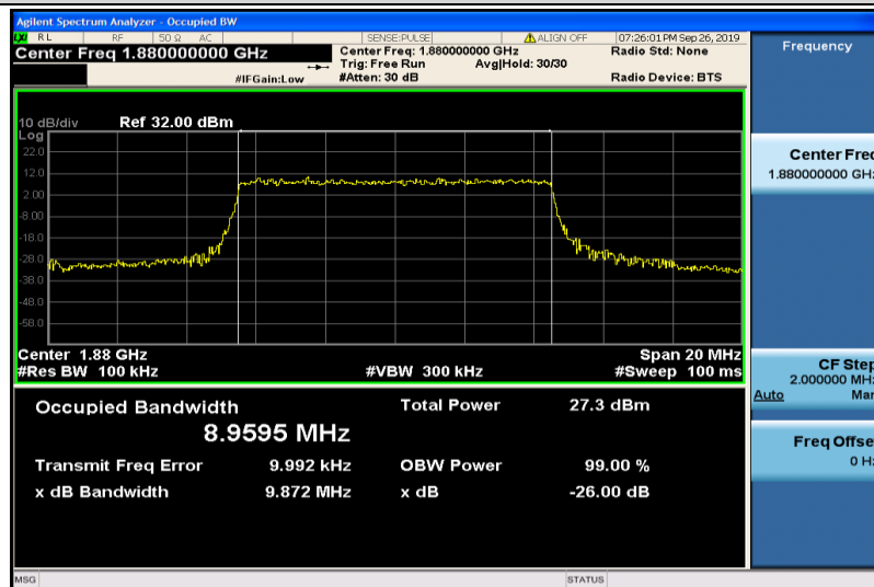
Band2-10MHz-16QAM-18900-50RB#0-8.9595
