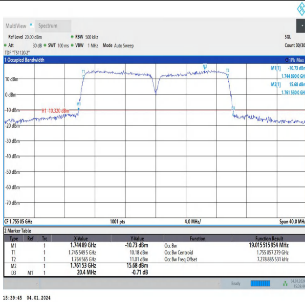
66-66-10MHz-10MHz-64QAM-64QAM-132373-132472-50RB#0-50RB#0-PASS
