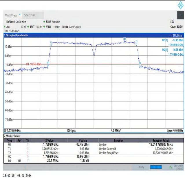
66-66-10MHz-10MHz-64QAM-64QAM-132523-132622-50RB#0-50RB#0-PASS
