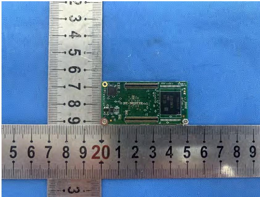
BT module:DART-6UL-5G
