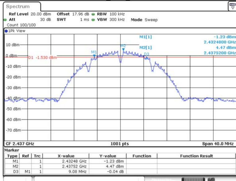
11B_Ant1_2437
