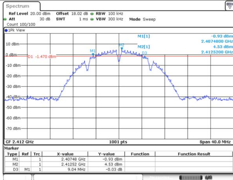
11B_Ant1_2412
