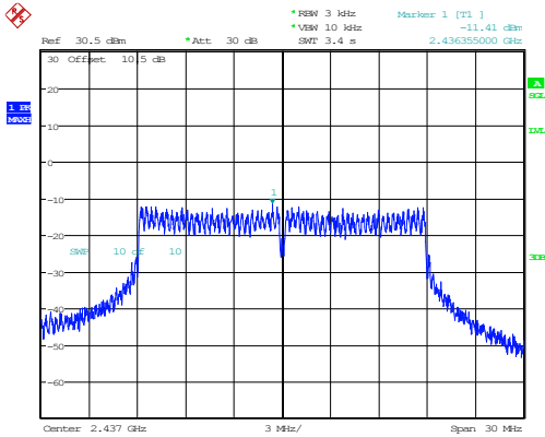
802.11n20_2437MHz_Chain 1
