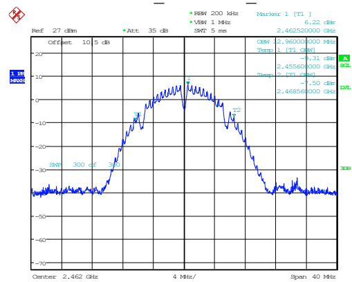
802.11b 2462MHz Chain 1
