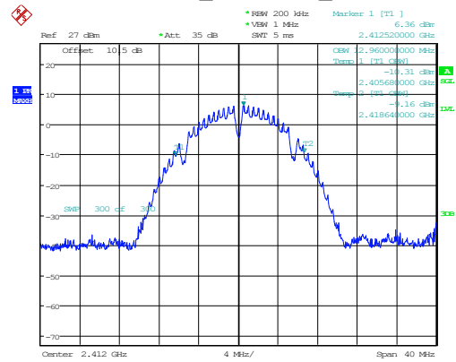
802.11b_2412MHz_Chain 1
