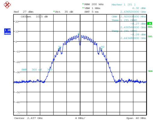
802.11b_2437MHz_Chain 0
