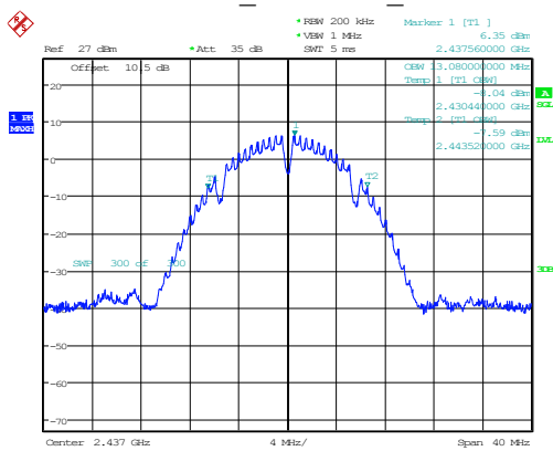
802.11b 2437MHz Chain 1
