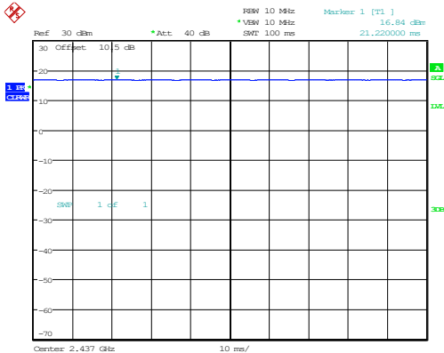
802.11b_2437MHz_Chain 0
