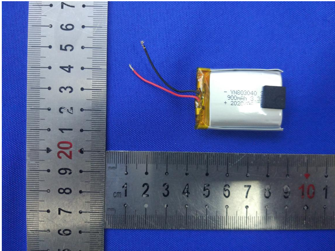
Model: WF80
