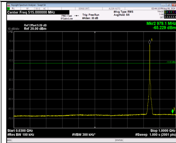
5-5-3MHz-5MHz-QPSK-QPSK-20586-20625-15RB#0-25 RB#0-30~1000MHz-PASS
