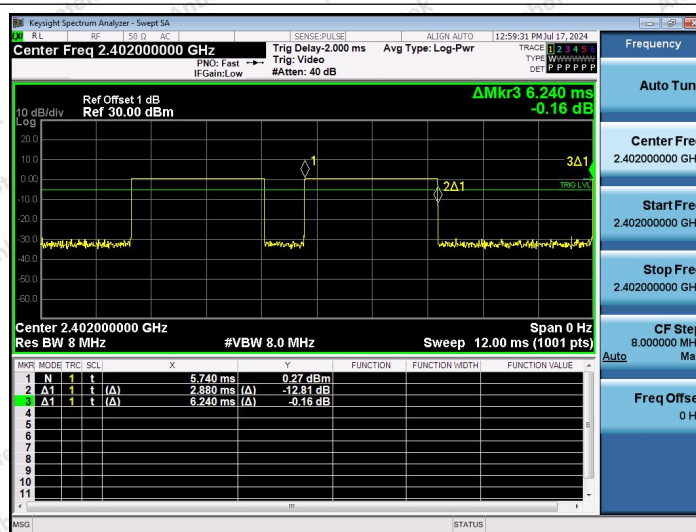
NTNV-2.4G-Ant1-2402
