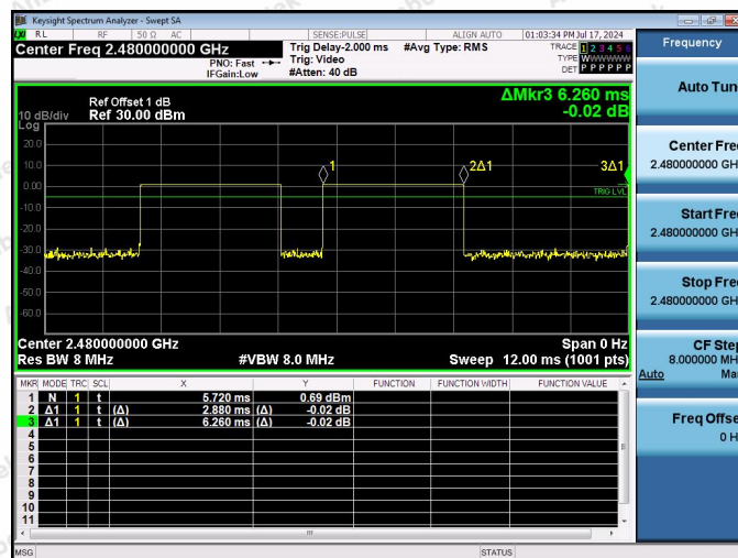
NTNV-2.4G-Ant1-2480
