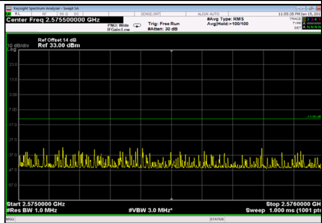
FDD07_5MHz_2567.5_QPSK_OneRB_low
