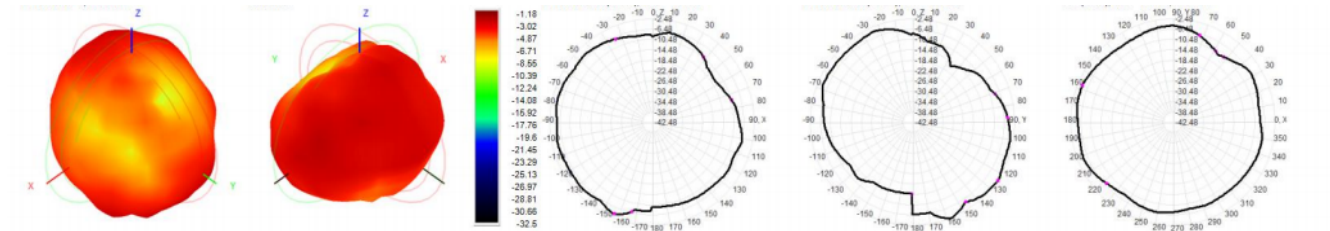
ANT2 5850MHZ
