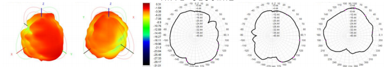
ANT1 5150MHZ
