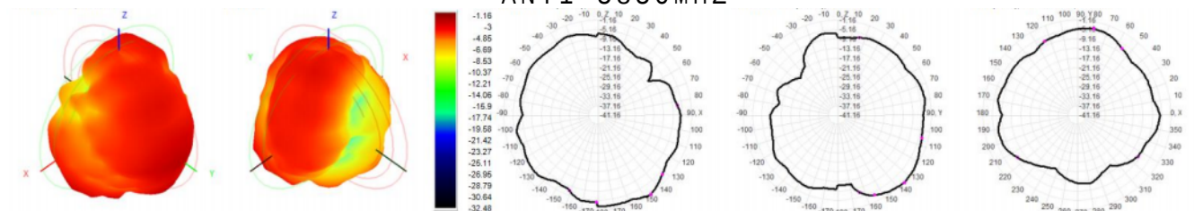
ANT1 5850MHZ
