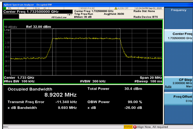
Band4-10MHz-QPSK-20175-50RB#0-8.9202
