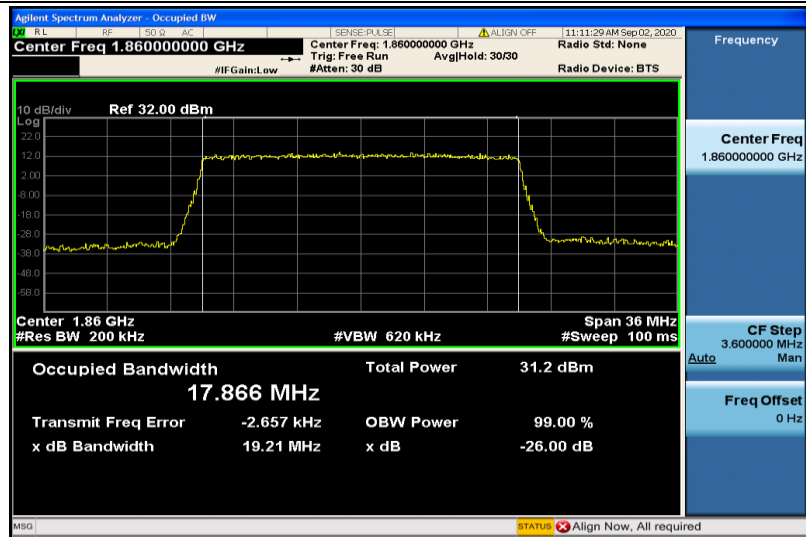
Band2-20MHz-QPSK-18700-100RB#0-17.866
