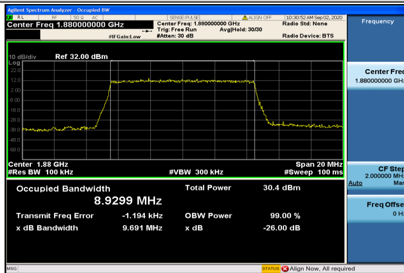
Band2-10MHz-QPSK-18900-50RB#0-8.9299
