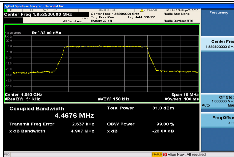
Band2-5MHz-QPSK-18625-25RB#0-4.4676
