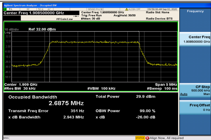
Band2-3MHz-QPSK-19185-15RB#0-2.6875
