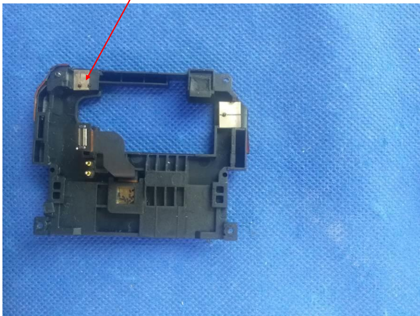
BLE Antenna
