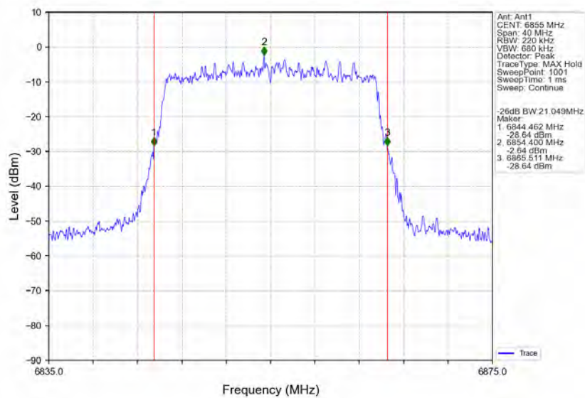
802.11ax(HE20)_HCH_6855MHz_RU242_Ant1_NTNV
