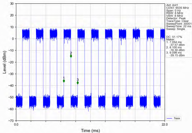
802.11ax(HE20)_LCH_6535MHz_RU242_Ant1_NTNV
