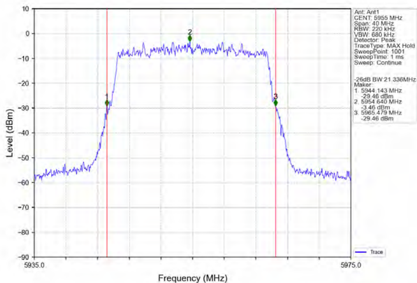
802.11ax(HE20)_LCH_5955MHz_RU242_Ant1_NTNV
