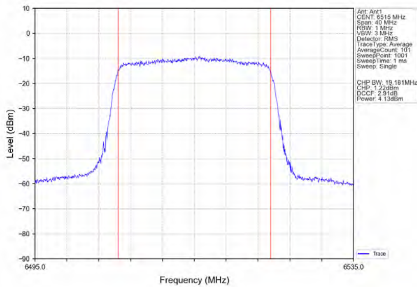
802.11ax(HE20)_HCH_6515MHz_RU242_Ant1_NTNV
