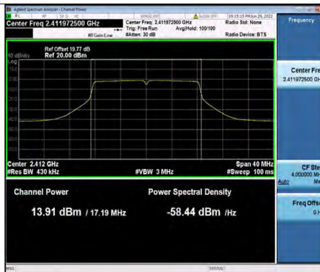
11G_Ant1_2412
