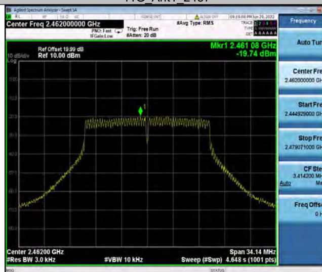
11G_Ant1_2462
