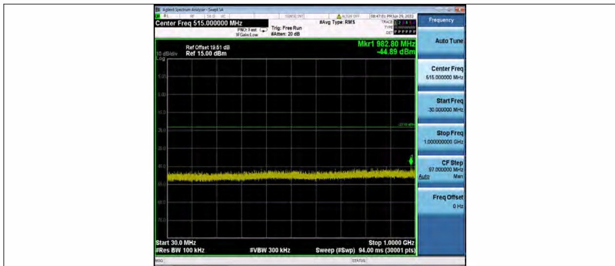
11B_Ant1_2412_30~1000
