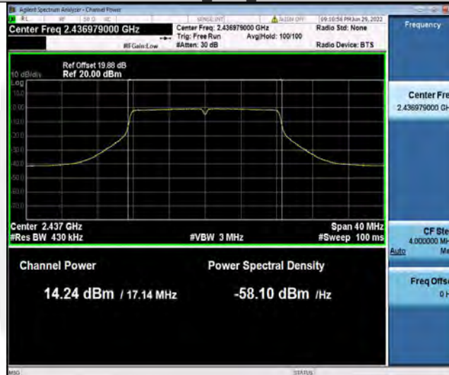
11G_Ant1_2437
