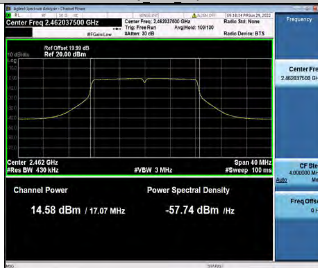
11G_Ant1_2462
