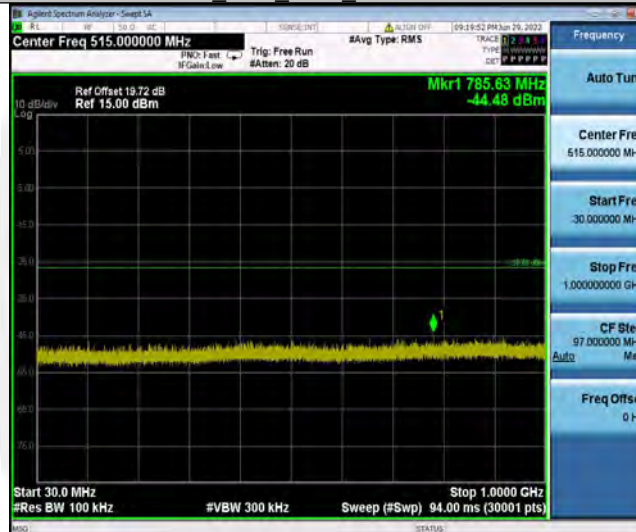
11G_Ant1_2462_30~1000
