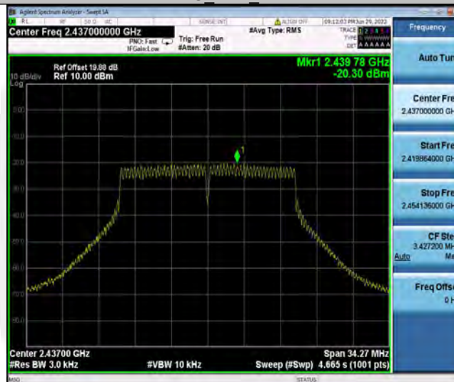
11G_Ant1_2437
