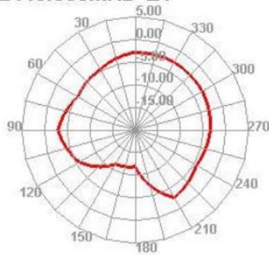
2440.000MHz E1
