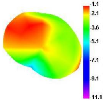
2440.000MHz E1
