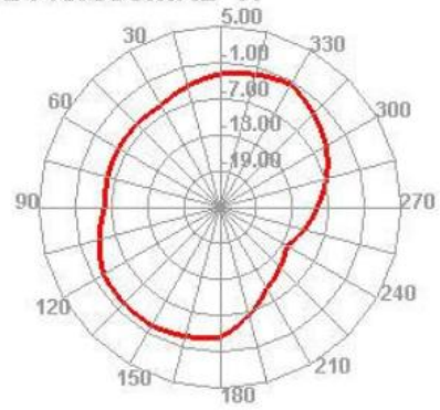
2440.000MHz E2
