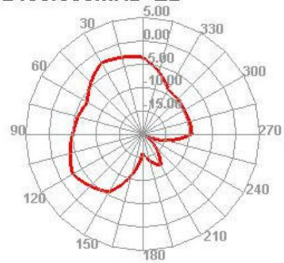
2400.000MHz E2
