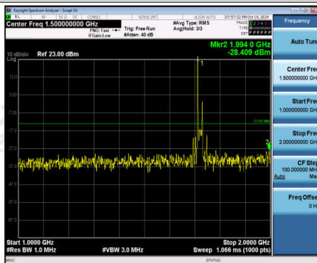
Band66-20MHz-QPSK-132072-1RB#0-Range2:1000~2000MHz
