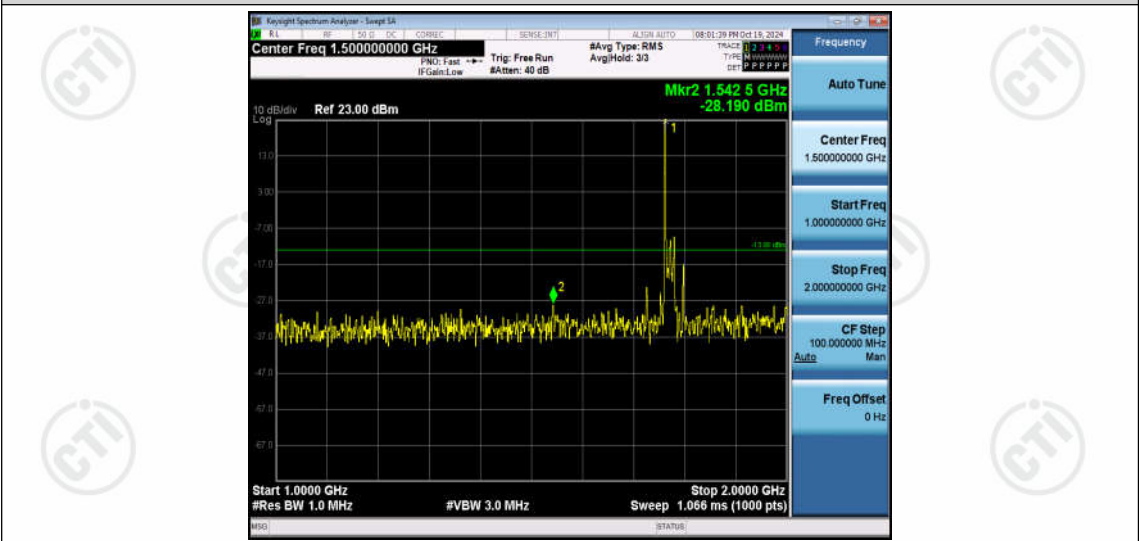
Band66-20MHz-QPSK-132572-1RB#0-Range2:1000~2000MHz
