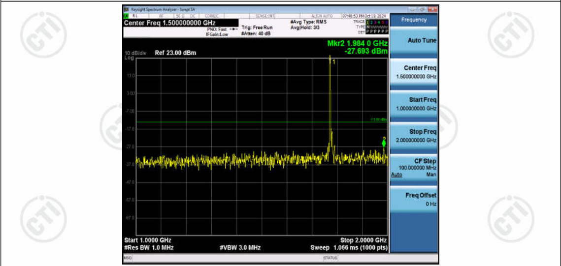
Band66-10MHz-QPSK-132622-1RB#0-Range2:1000~2000MHz
