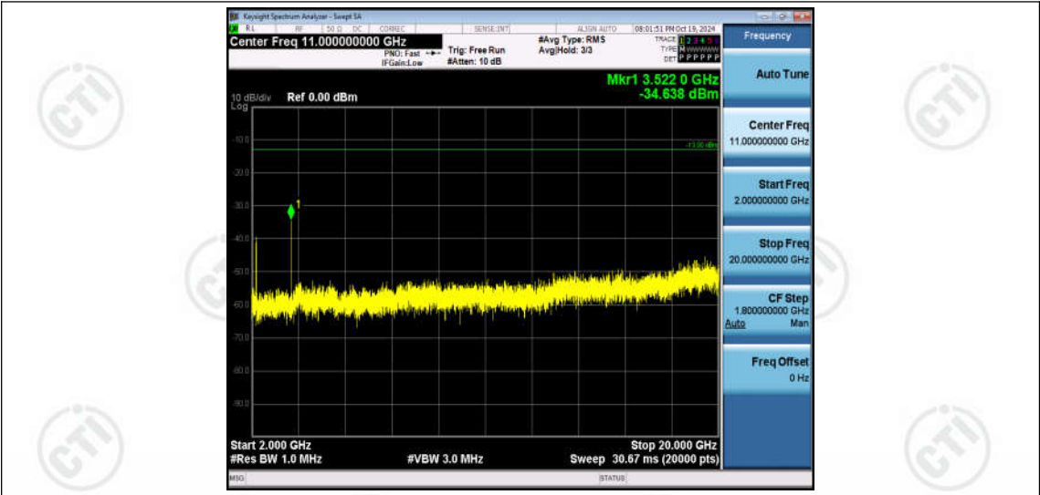
Band66-20MHz-QPSK-132572-1RB#0-Range3:2000~20000MHz
