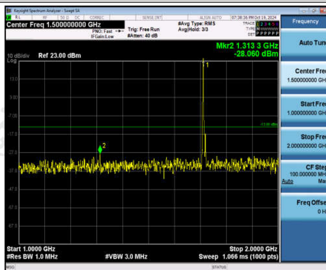
Band66-5MHz-QPSK-131997-1RB#0-Range2:1000~2000MHz
