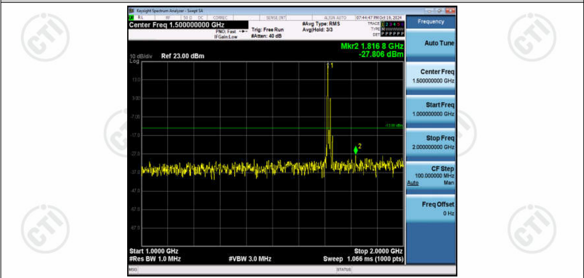
Band66-10MHz-QPSK-132022-1RB#0-Range2:1000~2000MHz
