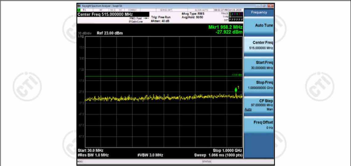
Band66-20MHz-QPSK-132572-1RB#0-Range1:30~1000MHz
