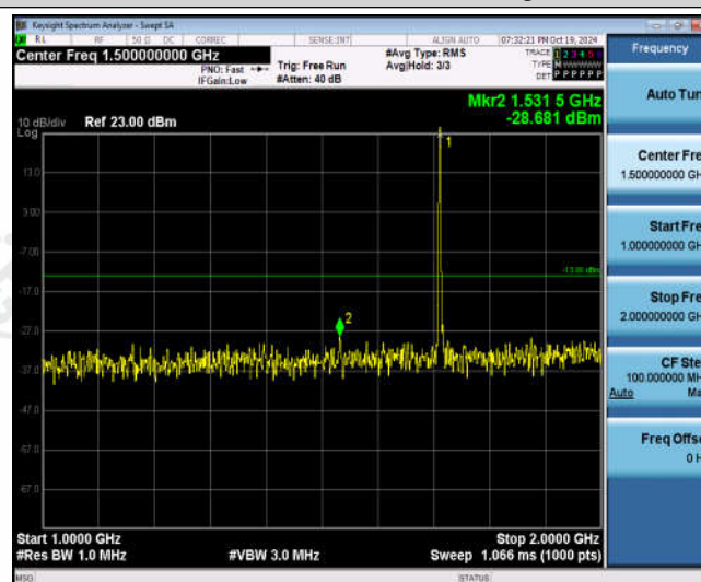
Band66-3MHz-QPSK-131987-1RB#0-Range2:1000~2000MHz
