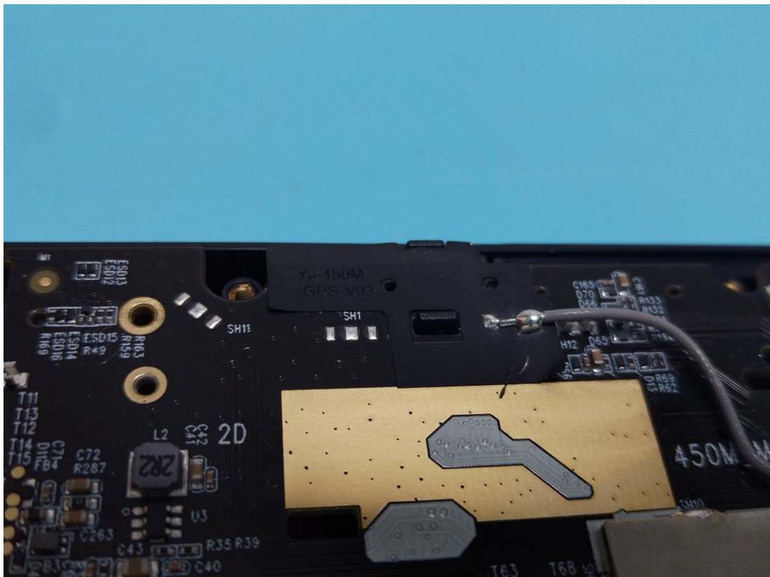
GPS ANT
