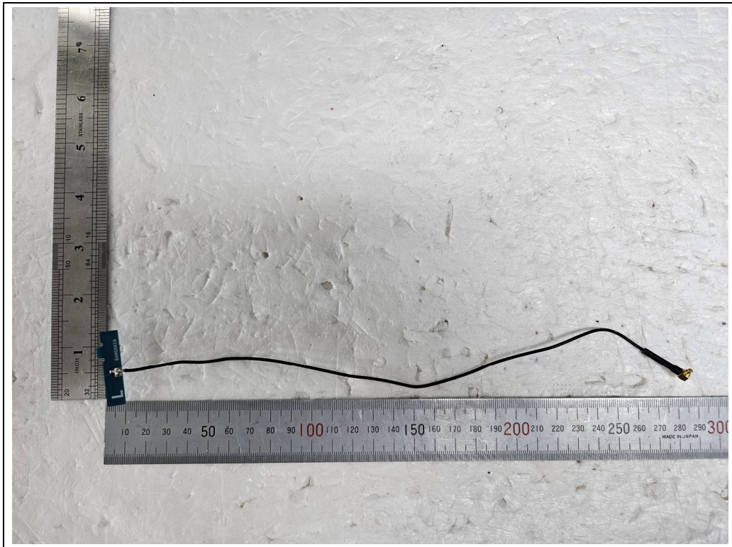
<2.4G, 5G WLAN Antenna>
