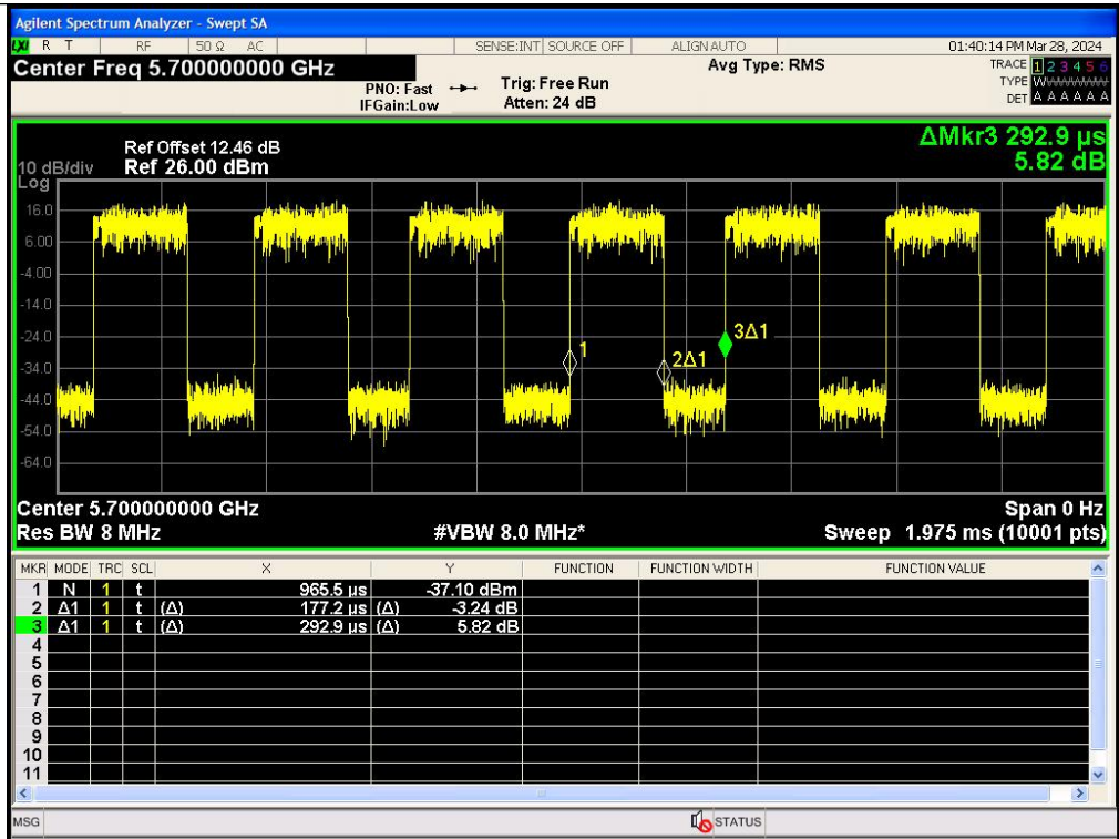
IEEE 802.11a_20MHz_Channel 140
