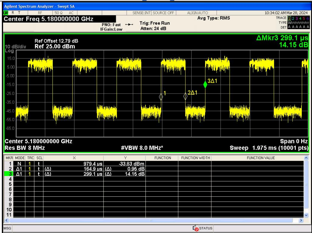
IEEE 802.11n_20MHz_Channel 36
